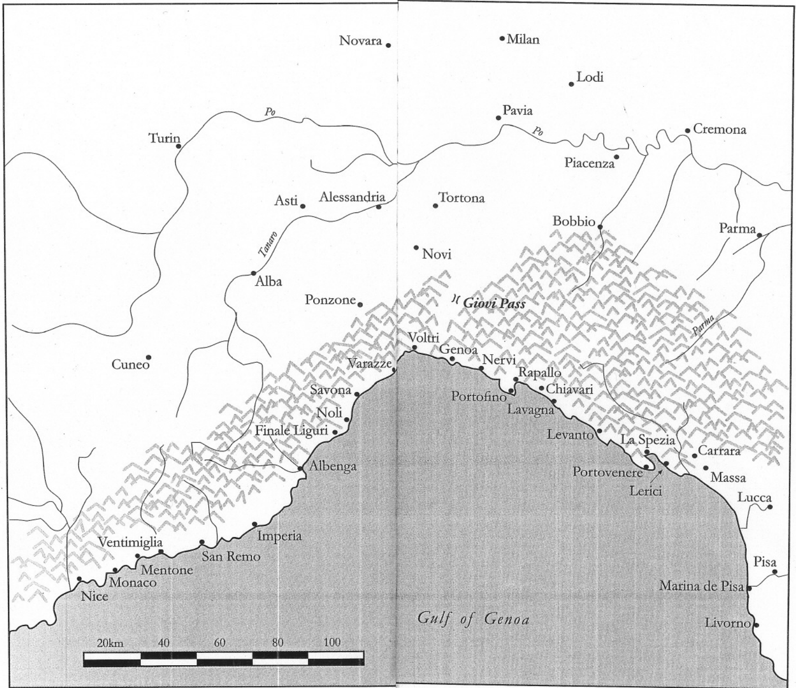
MAP 2. Liguria
